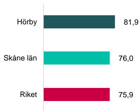
Figur 14 - Demografisk försörjningskvot, 2018
